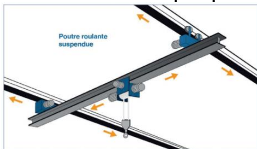
Poutre roulante suspendue
